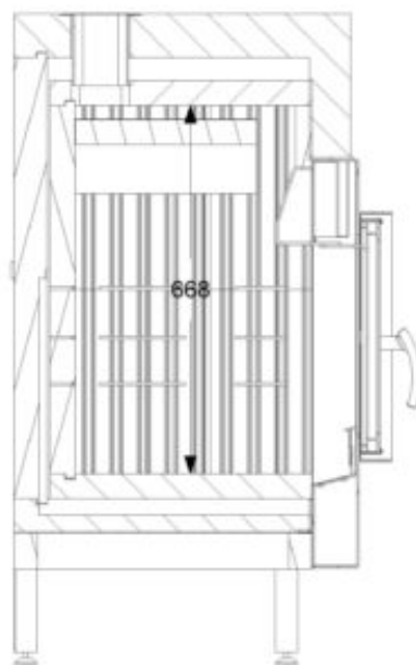
Przekrój B-B SKALA 1 : 10
