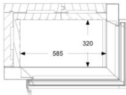
Przekrój A-A SKALA 1 : 10
