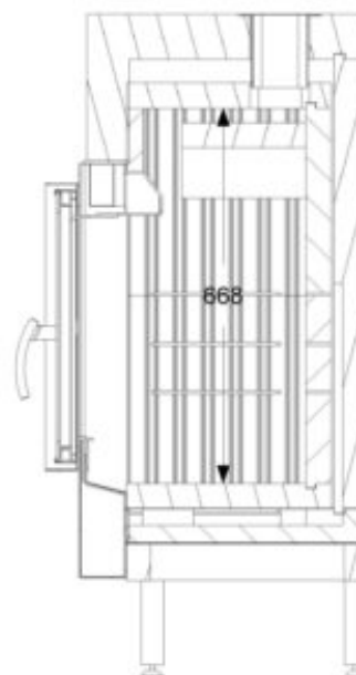
Przekrój B-B SKALA 1 : 10
