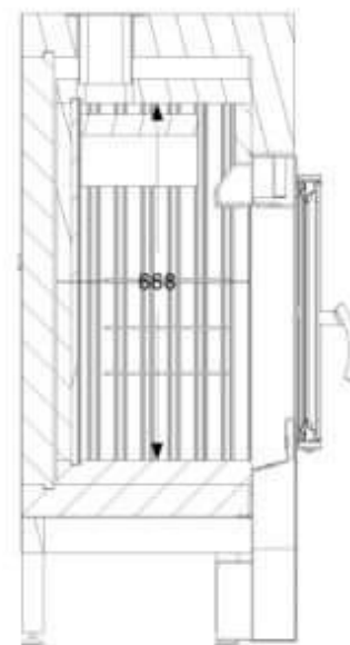
Przekrój B-B SKALA 1 : 10
