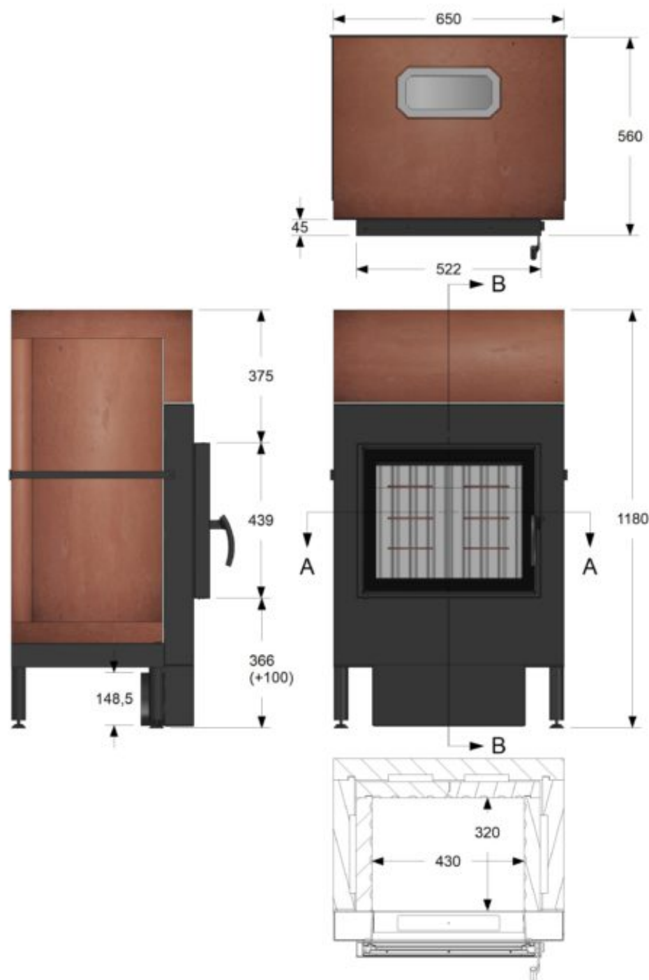
Przekrój A-A SKALA 1 : 10
