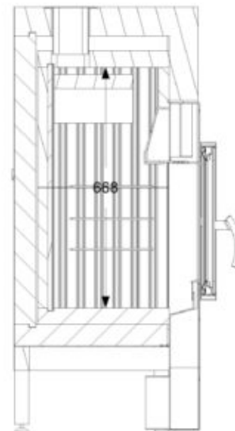
Przekrój B-B SKALA 1 : 10
