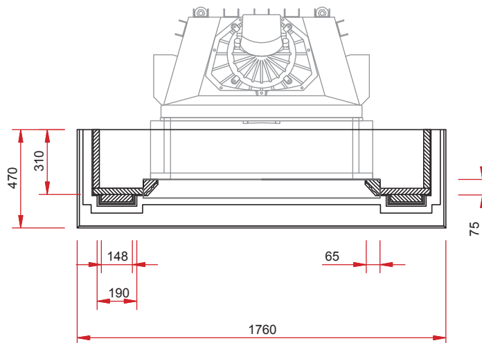
Draufsicht M 1:25
